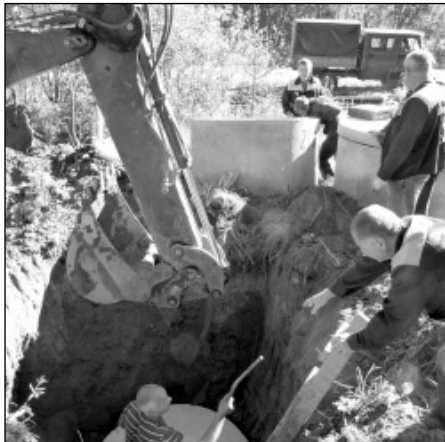
Специалисты Износковского участка ВКХ ГП «Калугаоблводоканал» ведут монтаж водопроводного колодца.
